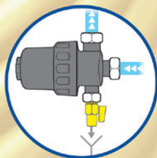
Installazione orizzontale con scarico basso
