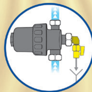
Installazione orizzontale con scarico laterale
